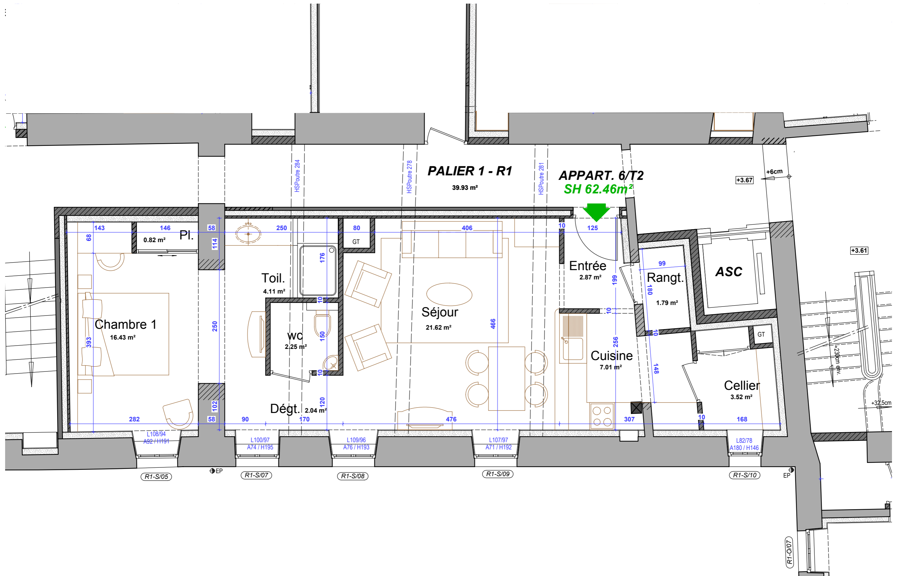
PLAN R1 - APPARTEMENT 6 - ECH. 1/50
