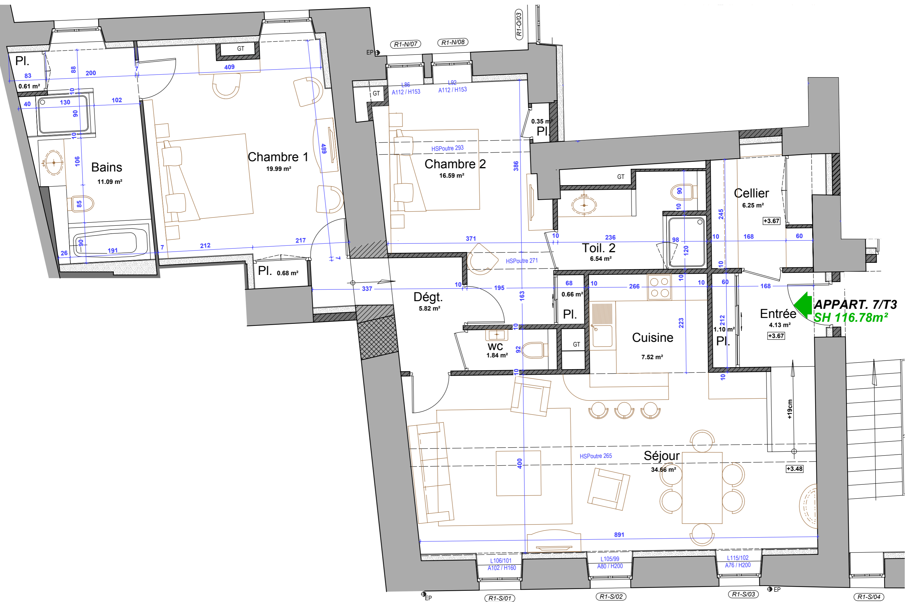
PLAN R1 - APPARTEMENT 7 - ECH. 1/50 11a
